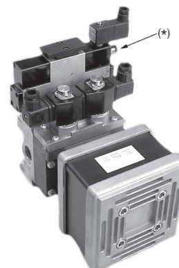
Com reset remoto (*) alimentação externa do reset
