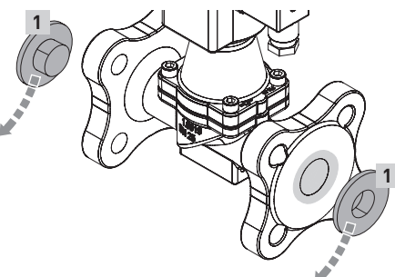
Schutzkrägen entnehmen
