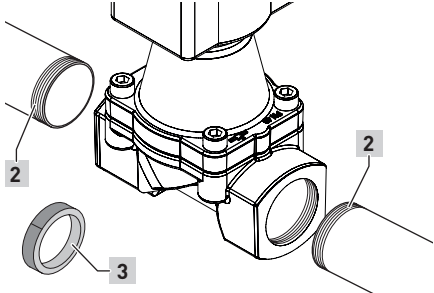
Gewinde der Rohrleitungen abdichten
