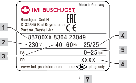
Leistungsschild (Beispiel)
