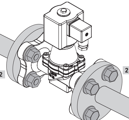
Rohrflansch mit Ventiflansch verbinden
