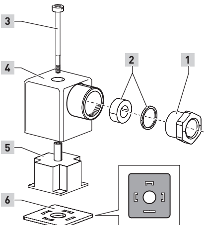
Übersicht: Gerätesteckdose
