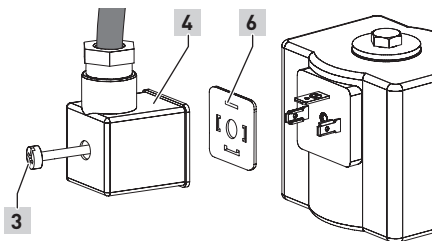
montierte Gerätesteckdose aufstecken
