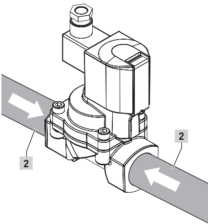
Rohrleitungen mit Ventil verbinden
