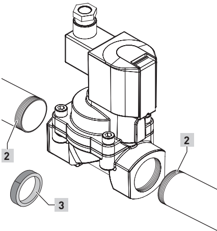
Gewinde der Rohrleitungen abdichten
