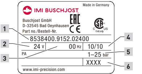
Leistungsschild (Beispiel)
