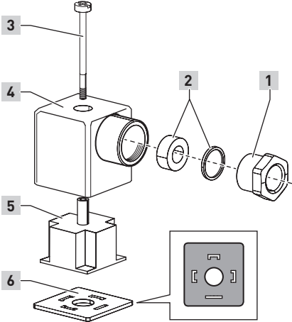
Übersicht: Gerätesteckdose
