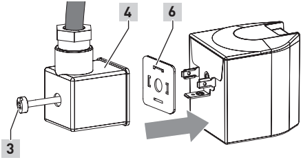
montierte Gerätesteckdose aufstecken
