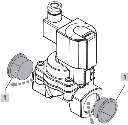
Verschlussstopfen entnehmen
