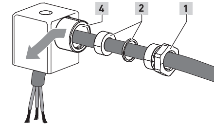
Kabel durch Gerätesteckdose führen
