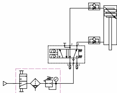
Przykłady funkcji bezpieczeństwa bezpieczne odpowietrzanie Kat. 4 PL-e
