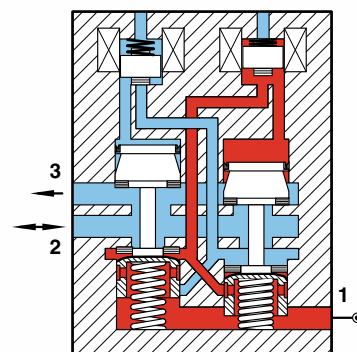
Port 2 odpowietrzony przez tłumik hałasu na porcie 3
