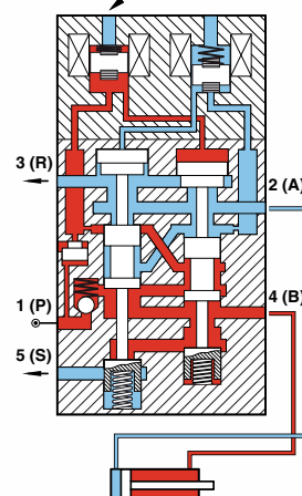
Położenie bezpieczne W przypadku niesymetrycznegoysterowania
