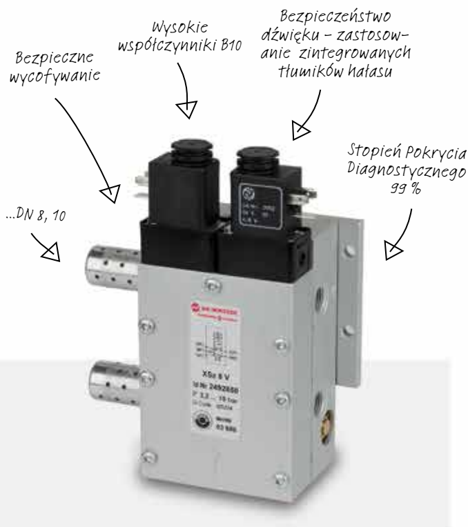
Przykłady funkcji bezpieczeństwa bezpieczne odpowietrzanie Kat. 4 PL-e
