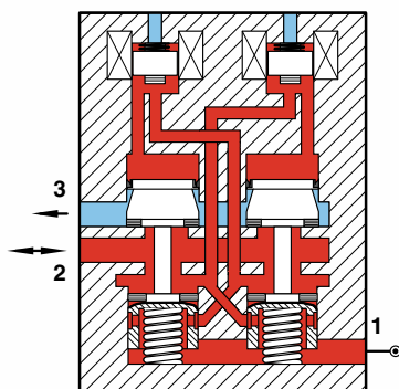
Ciśnienie z portu 1 przekazane do portu roboczego 2
