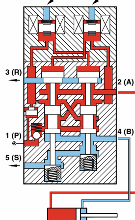
Położenie robocze Obie cewki zasilane
