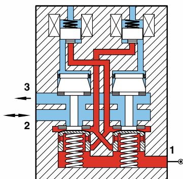
Port 2 odpowietrzony przez tłumik hałasu na porcie 3
