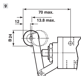
Roleta alavanca – G1/4
