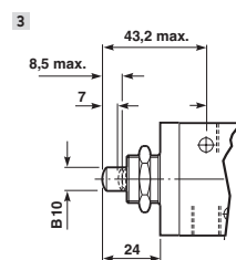
Botão palma – G1/4
