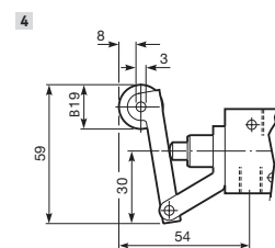
Roleta Alavanca – G1/8
