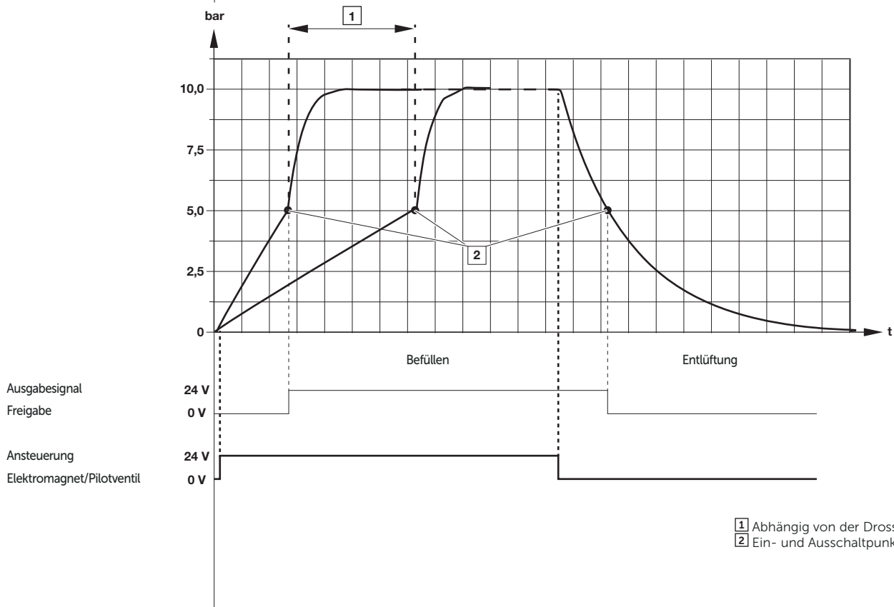
Schaltverhalten bei 10 bar Versorgungsdruck (PVer)
